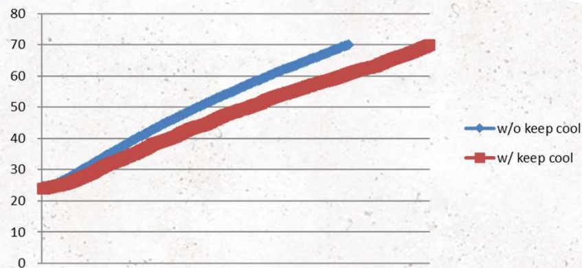
Curva de temperatura de 18 V y 2,0 Ah
